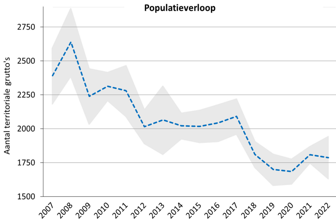
Figuur 3.1.1: Verloop van het aantal territoriale grutto's in het studiegebied met in grijs de foutmarge op basis van verschillen in tellingen en geschatte waarden.
