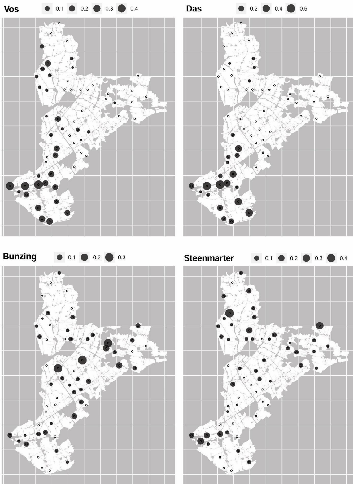
Figuur 3.2.2: Gemiddelde aantallen (zwarte cirkels naar grootte) door cameravallen geregistreerde waarnemingen per dag van vos, das, bunzing en steenmarter op vaste locaties (toegangsdammen) in het studiegebied in 2022. Open cirkels geven de cameralocaties aan waar de soort niet werd geregistreerd.
