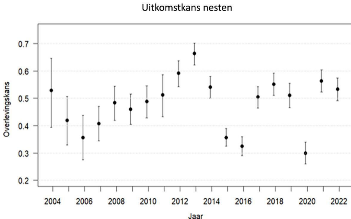
Figuur 3.1.3: Uitkomstkansen van nesten gebaseerd op een nest-overlevingsanalyse waarmee rekening wordt gehouden dat nesten al kunnen zijn gepreedeerd voordat ze gevonden worden. Een overlevingskans van 1 komt overeen met 100%.
