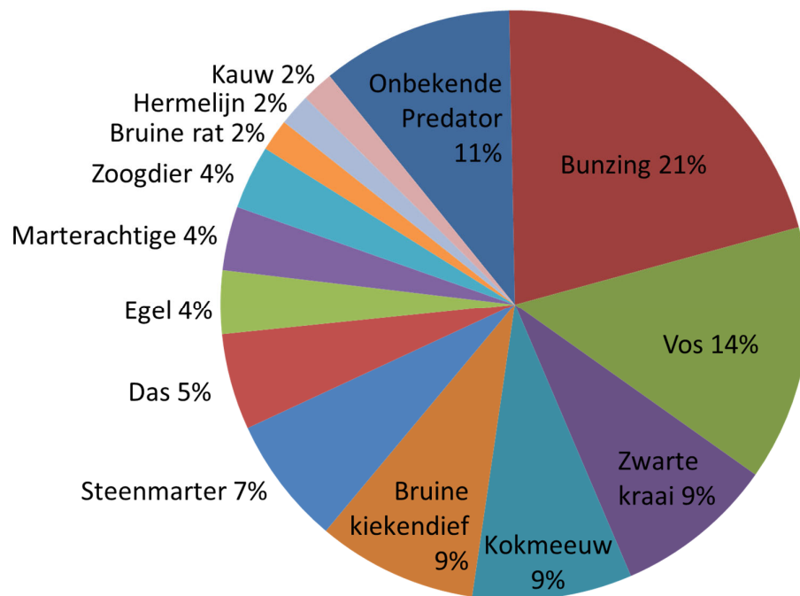
Figuur 3.1.9: De verschillende soorten predatoren verantwoordelijk voor nestpredatie van 57 van de 212 met cameraval gevolgte gruttonesten. In sommige gevallen ('onbekende predator') kon geen predator worden vastgesteld (b.v. door hoog gras).
