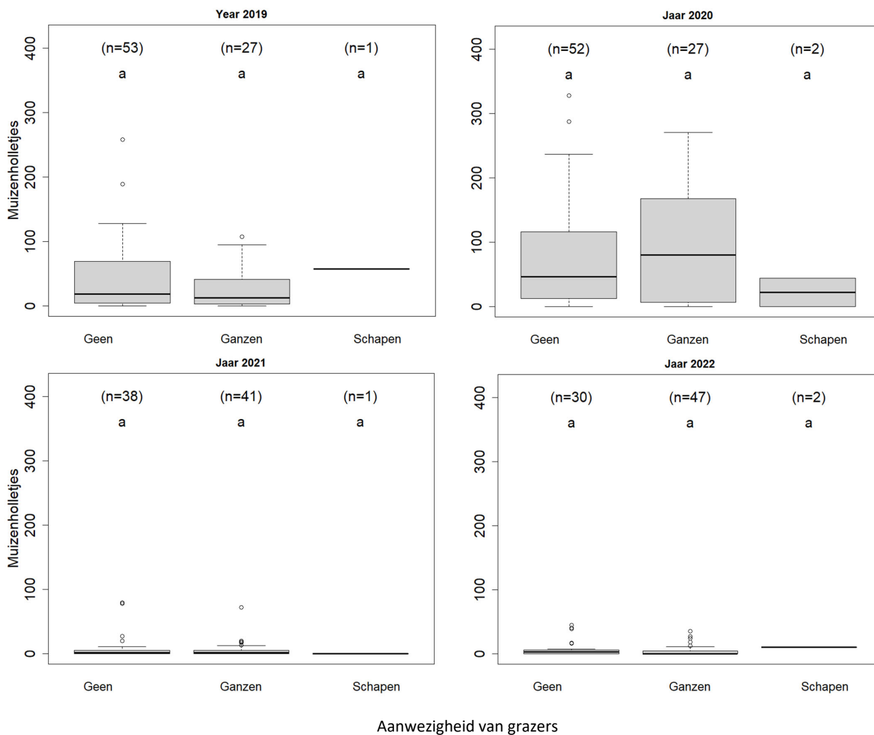
Figuur 3.2.6: Verdeling van aantallen muizenholletjes in relatie tot de aan- of afwezigheid van grazers. Er werden geen significante verschillen gevonden.
