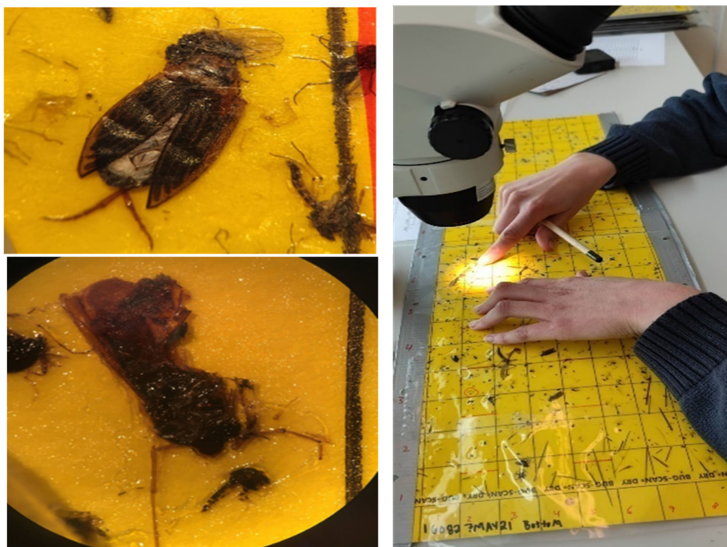
Figuur 3.3.1: Linksboven en -onder foto's van insecten op de plakval. Rechts een foto van hoe stuk voor stuk de insecten worden bekeken, geteld, gemeten en geïdentificeerd.
