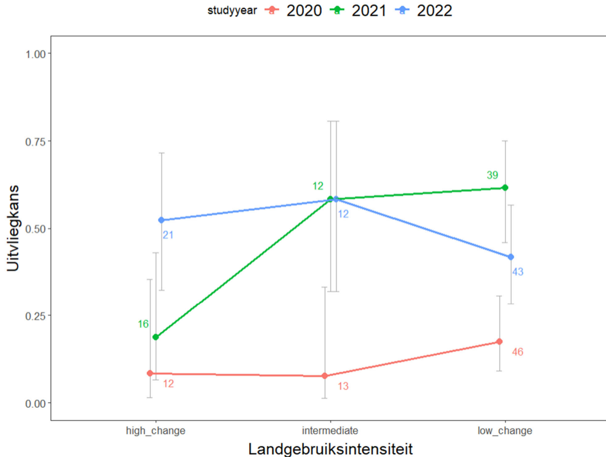
Figuur 3.1.14: De uitvliegkans van met radiozenders gevolgte families in 2020 (rood), 2021 (groen) en 2022 (blauw) afhankelijk van de landgebruiksintensiteit van het weiland waar de kuikens uit het ei kwamen. Gemiddelden per landgebruiksintensiteit-categorie zijn uitgezet met 95% betrouwbaarheidsintervallen. Getallen naast de datapunten zijn de steekproefgroottes.
