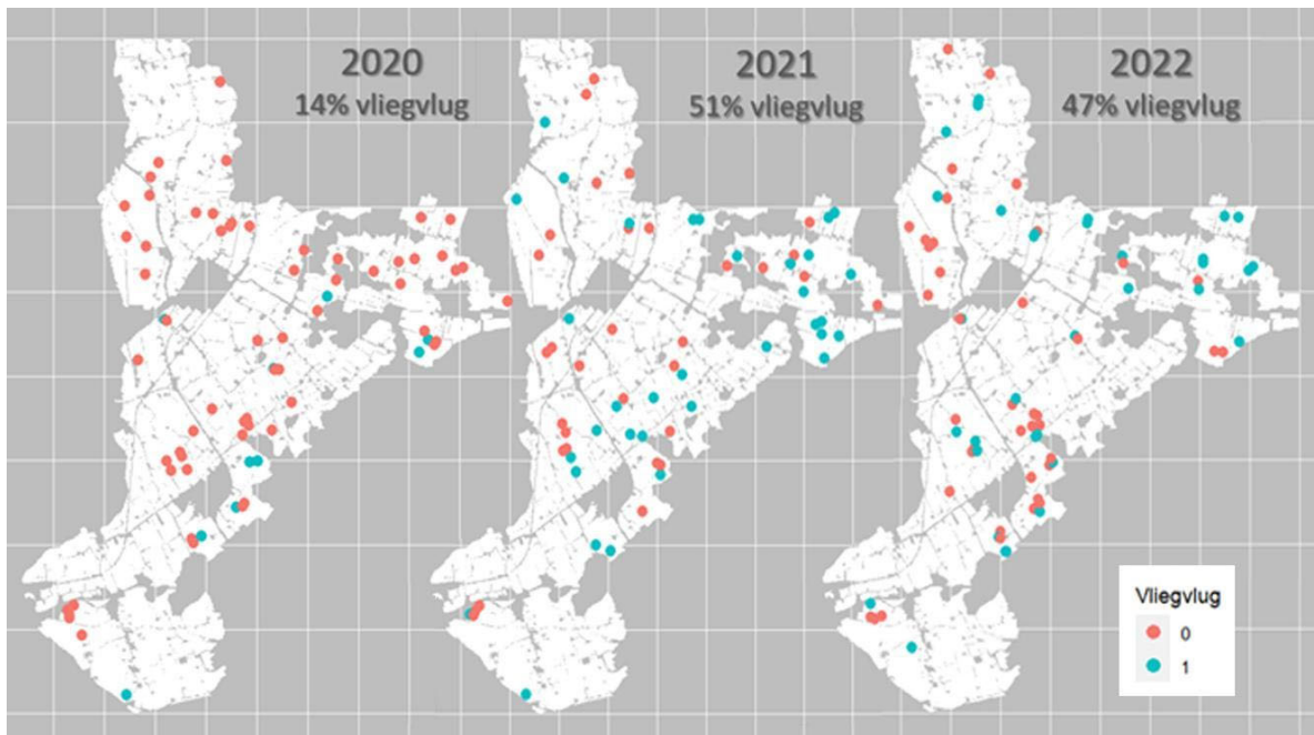
Figuur 3.1.13: Het uitvliegsucces van de met radiozender gevolgde families in het studiegebied in 2020 t/m 2021. Rood (0) = geen van de kuikens werd vliegvlug en blauw (1) = minstens één van de kuikens werd vliegvlug.
